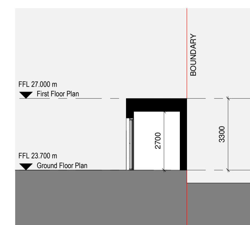
A Cross Section AA 1 : 100
