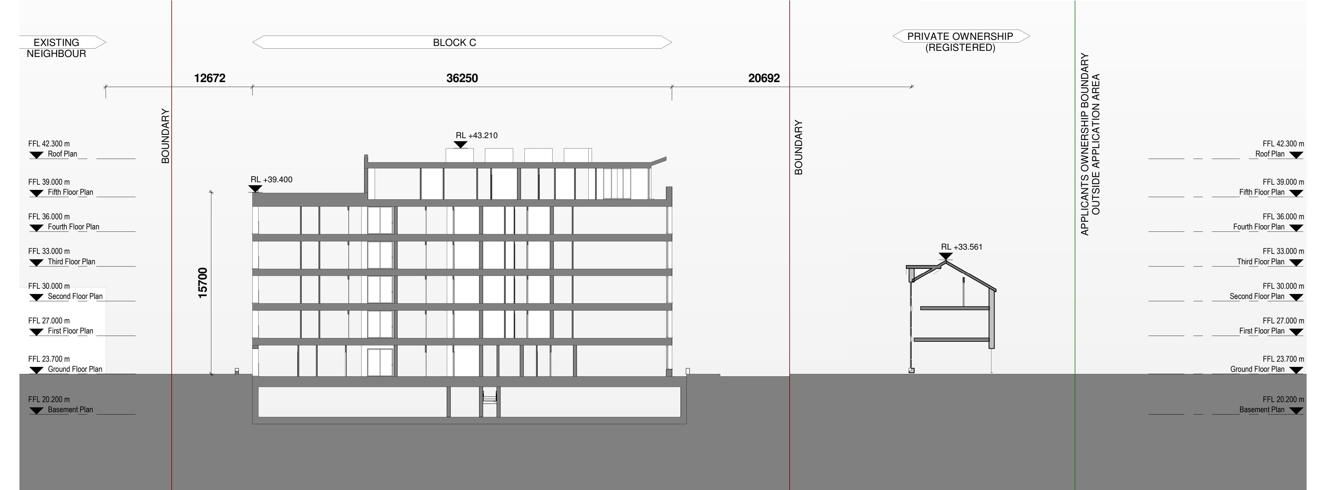
D Contextual Site Section DD 1 : 200
