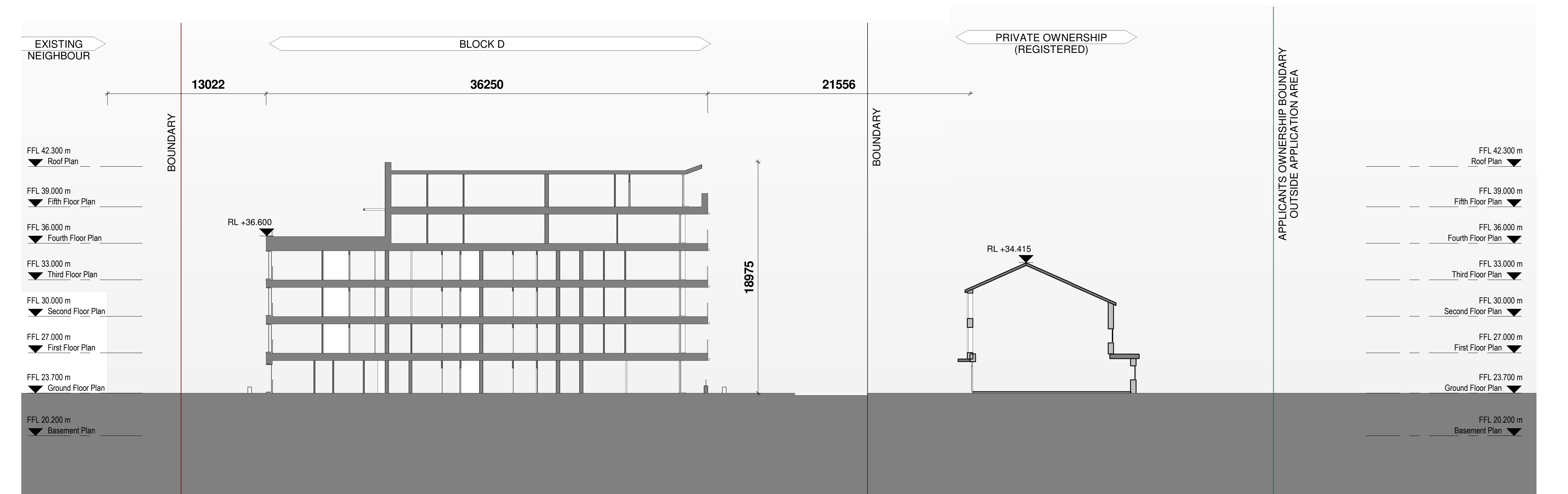
F Contextual Site Section FF 1 : 200
